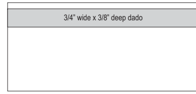
Top Return (Qty: 2)- 3"=1'-0"
